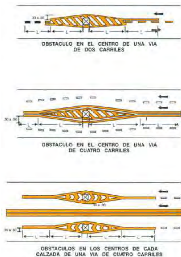
FIGURA 3.2.8.01 EJEMPLOS TÍPICOS DE LA DEMARCACIÓN DEL PAVIMENTO EN CASO DE OBSTÁCULOS DENTRO DE LA VÍA (Ej. CASSETAS DE PEAJE)
