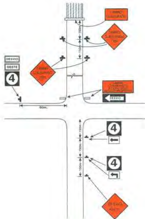
FIGURA 4.2.3.03 EJEMPLO TIPICO DE SEÑALIZACION PARA EL CASO DE DESVIAR E TRANSITO ANTES DE LA ZONA EN CONSTRUCCION
