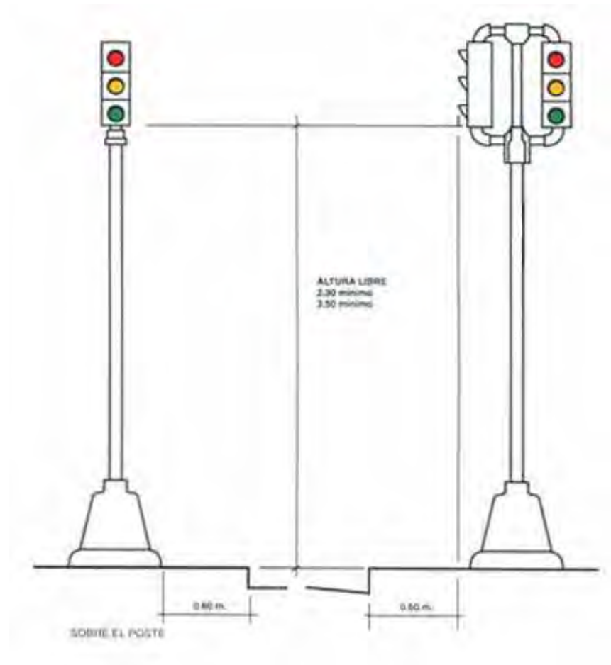
FIG. 5.4 SEMAFOROS MONTADOS EN POSTES
