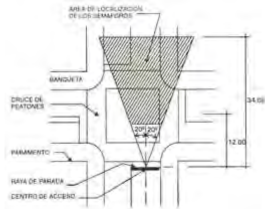
FIG. 5.3 LOCALIZACION DE LAS CARAS DEL SEMAFORO EN EL LADO MAS LEJANO DEL ACCESO DE LA INTERSECCION
